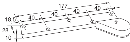
9143DS(L) Offset Door strap
