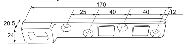
9123 Door strap
